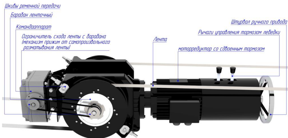
Рисунок 2.2 – Внешний вид лебедки ленточной
